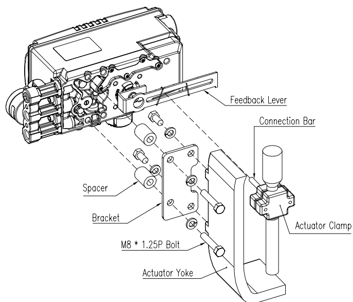
图3-4: 直行程定位器, 支架, 执行器
