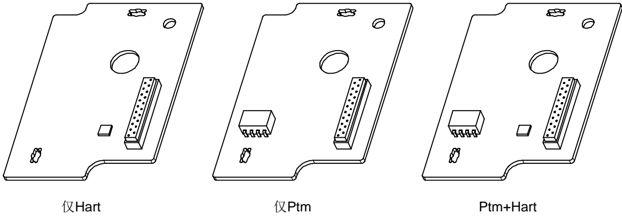
图7-1: 三种的副PCB
