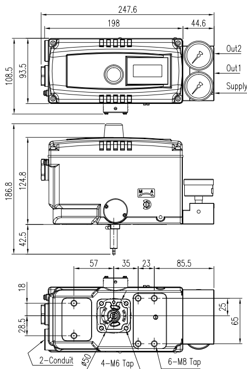
图 2-7: YT-3750R+LS
