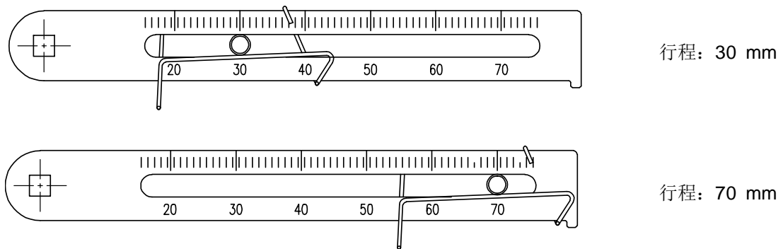
图3-14: YT-3702L反馈杆和连接杆的位置
