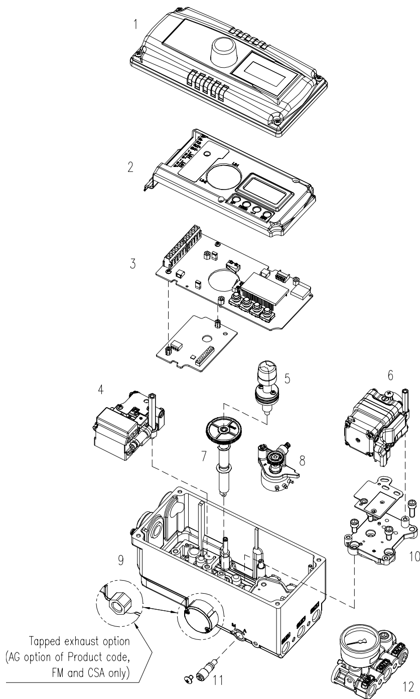
图2-2: 限位开关型定位器分解图
