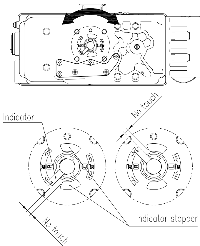
图3-23: 指标不得触及阀门行程0 % ~ 100 %处的指标止动件
