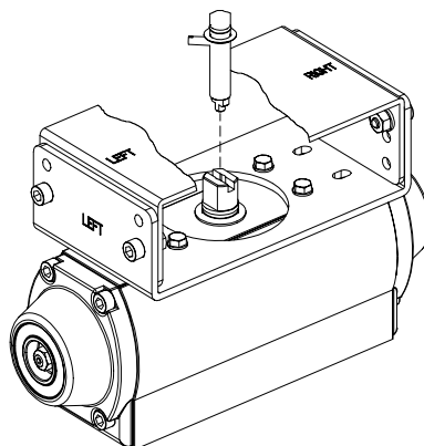
图3-22: 主轴中心对齐
