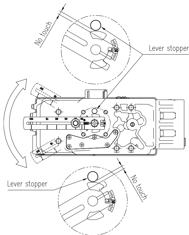
图3-15: YT-3700L / 3750L反馈杆不得触及阀门行程0% ~ 100%处的止动件。
