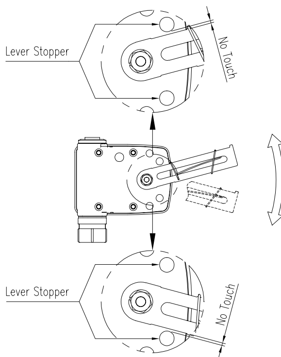
图3-16: YT-3702L反馈杆不得触及阀门行程0 % ~ 100 %处的止动件。
