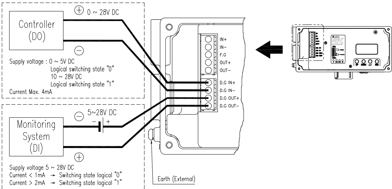
图5-2: 端子概览 2
