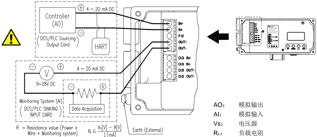
图5-1: 端子概览 1
