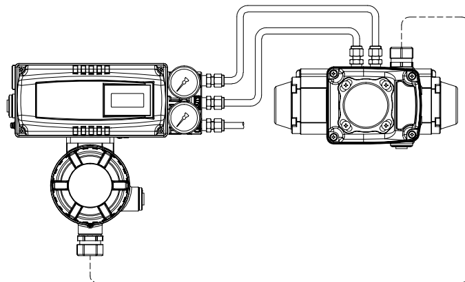
图4-8: 双作用角行程执行器(YT-3702R)
