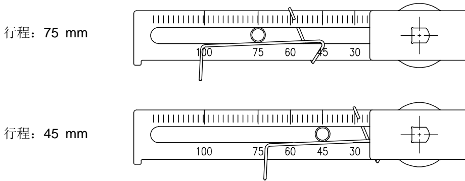
图3-13: YT-3700L / 3750L反馈杆和连接杆的位置
