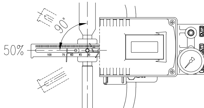
图3-11：YT-3700L / 3750L反馈杆和阀杆
