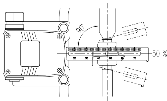
图3-12：YT-3702L反馈杆和阀杆
