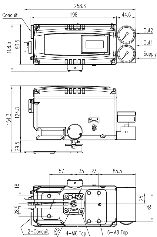
图 2-6: YT-3750L
