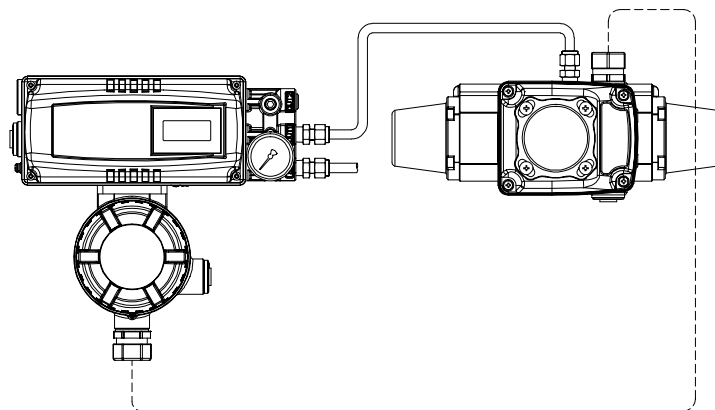
图4-4: 单作用角行程执行器(YT-3702R)
