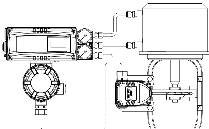
图4-7: 双作用直行程执行器(YT-3702L)
