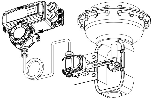
图3-3: YT-3702直行程定位器安装示例
