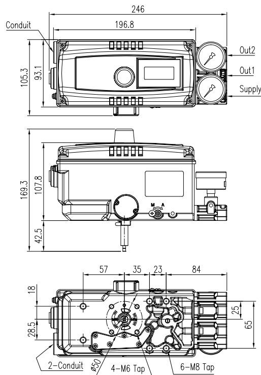
图 2-5: YT-3700R+LS
