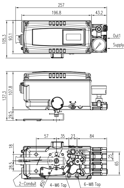
图 2-4: YT-3700L
