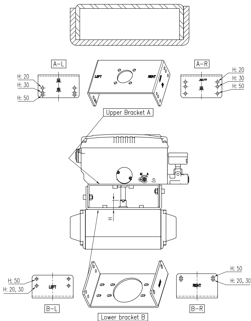
图3-19: 支架和定位器
