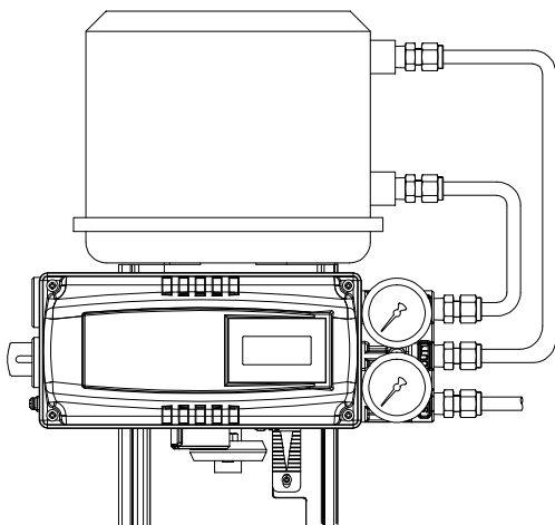
图4-5: 双作用直行程执行器(YT-3700L / 3750L)
