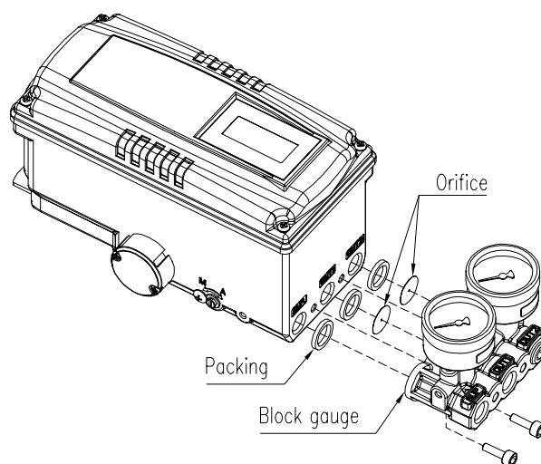
图6-4: 孔口件安装
