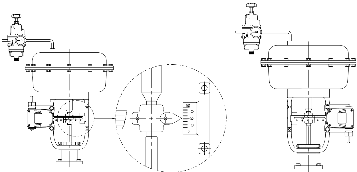
图3-8: 将YT-3702L安装到执行器的左轭上
