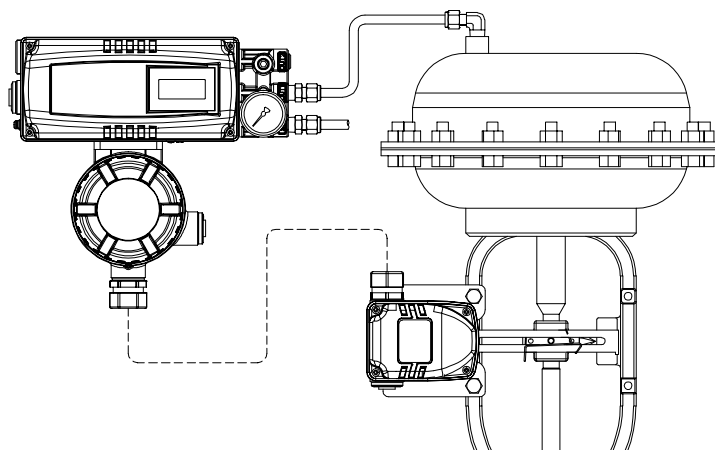
图4-3: 单作用直行程执行器(YT-3702L)
