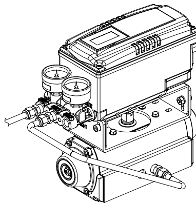
图4-2: 单作用角行程执行器(YT-3700L / 3750L)
