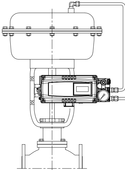
图3-2: YT-3700 / 3750直行程定位器安装示例
