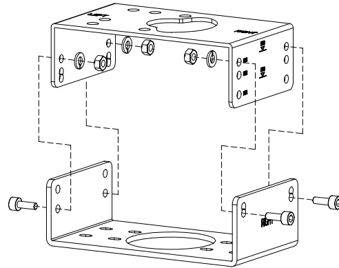
图3-21: 支架分解图
