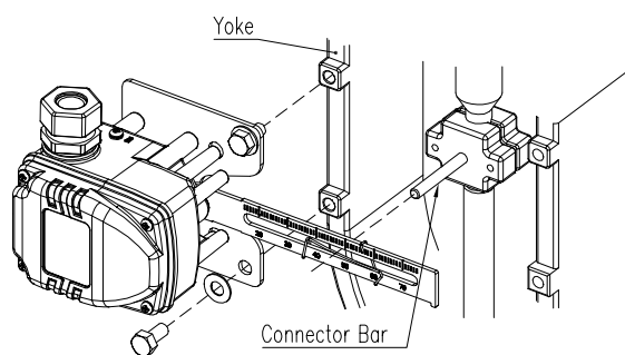
图3-6: 将支架安装于执行器轭上 (YT-3702L)
