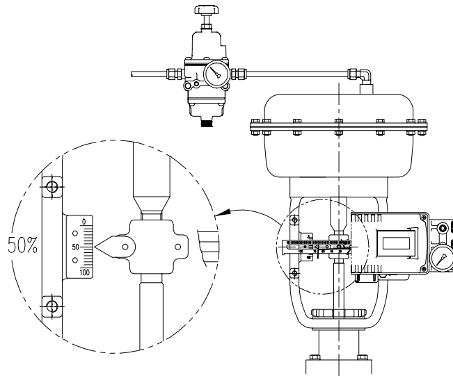
图3-7: YT-3700L / 3750L
