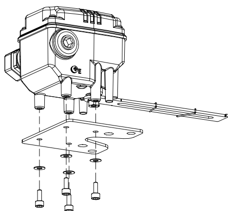
图3-5: 将定位器安装于支架上(YT-3702L)
