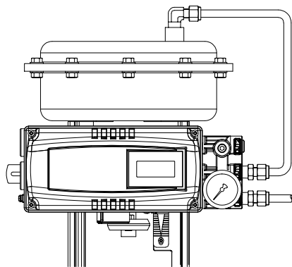
图4-1: 单作用直行程执行器(YT-3700L / 3750L)
