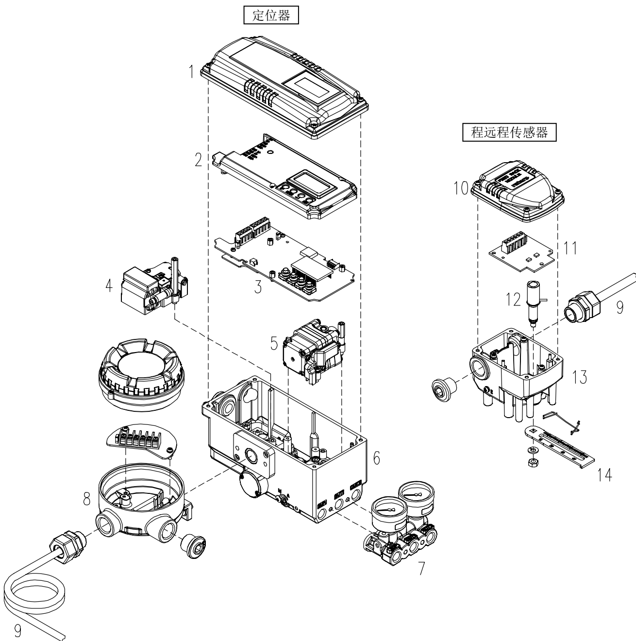
图2-3: YT-3301分解图
