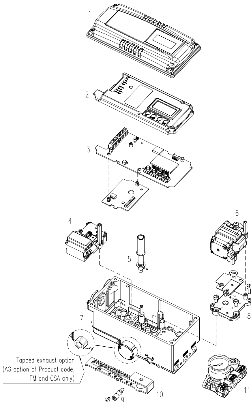
图2-1: 标准型定位器分解图
